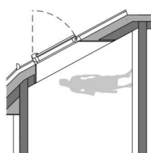
SCHNITT A
