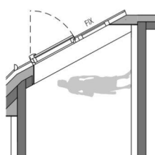
SCHNITT B
