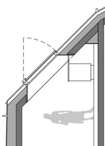
SCHNITT E
