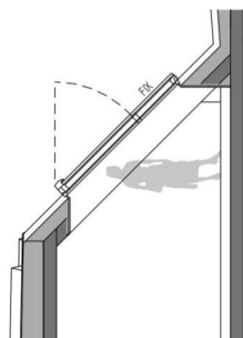
SCHNITT B
