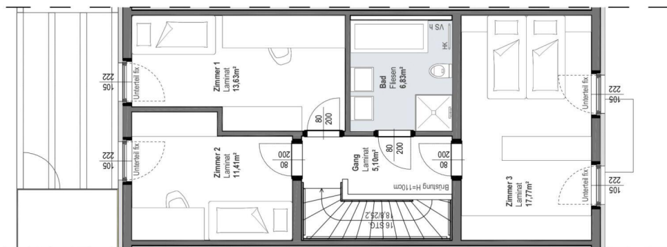
OBERGESCHOSS
