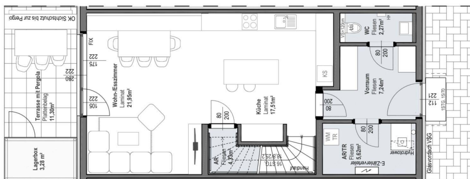
ERDGESCHOSS
