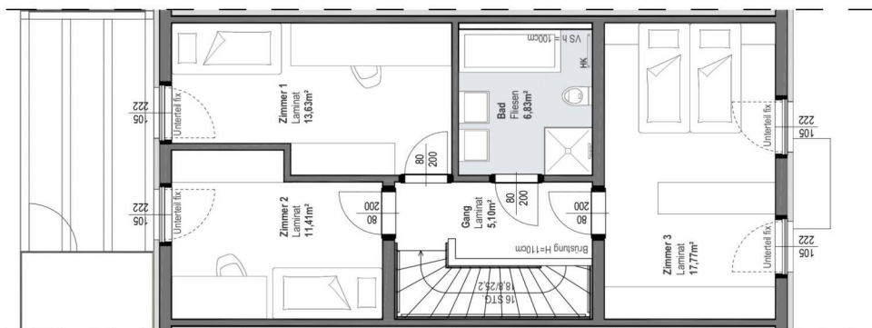
OBERGESCHOSS
