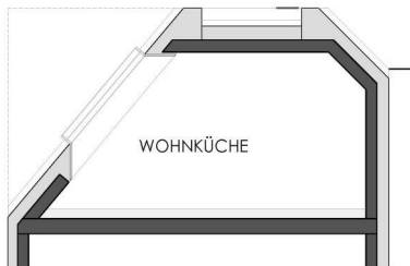
Klappschnitt 12 - Wohnküche
