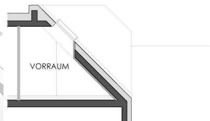
Klappschnitt 12 - Vorraum
