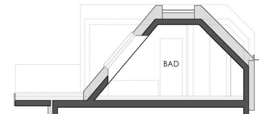
Klappschnitt 12 - Bad
